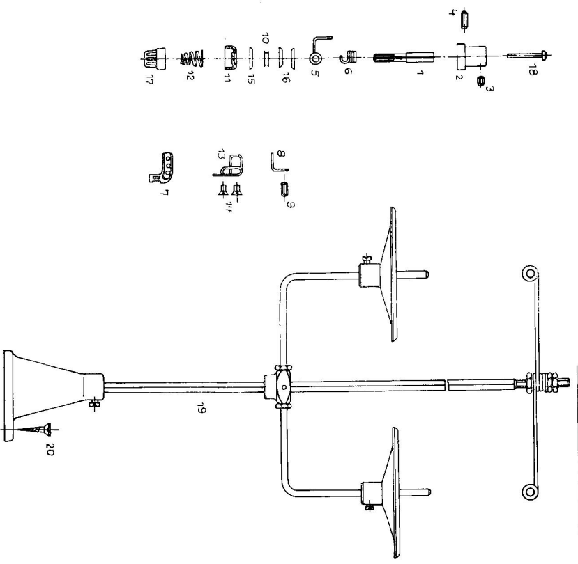
Tafel 7 Fodenspanner
