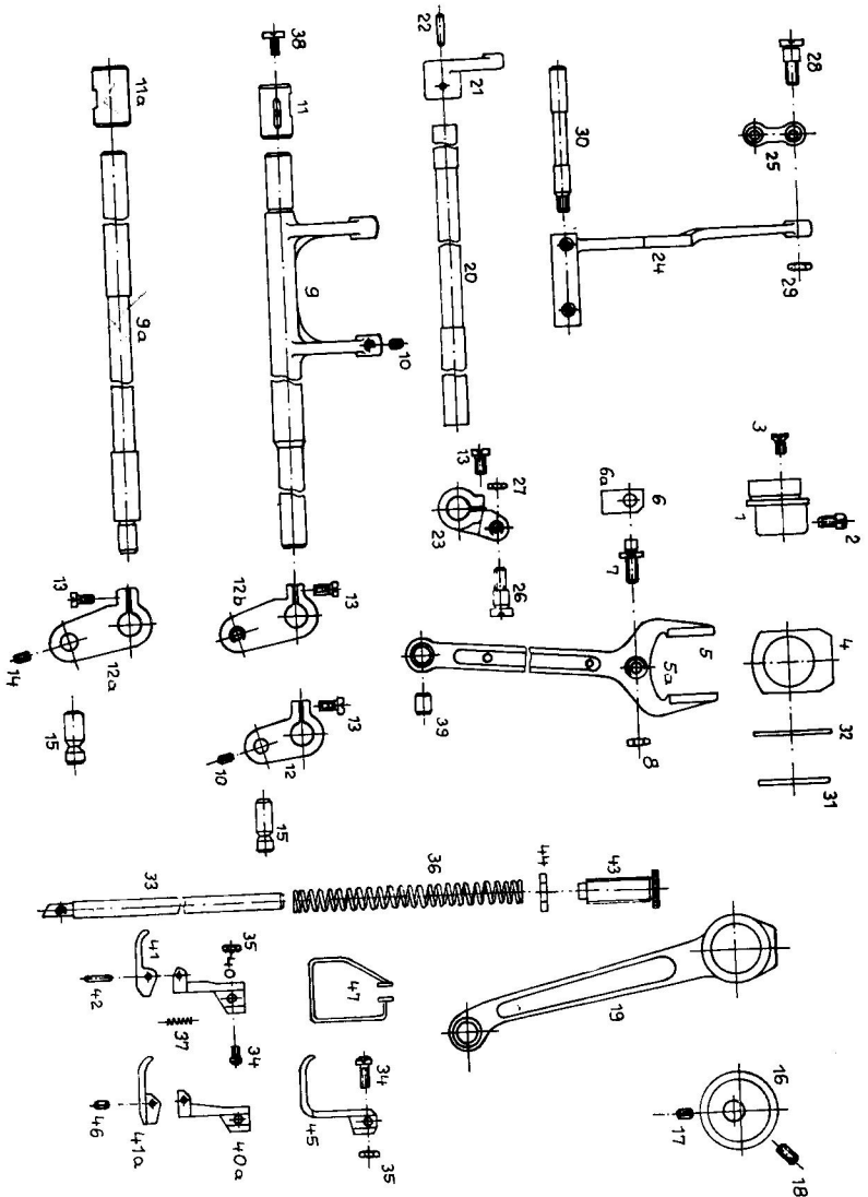
Tafel 4 Transporteurmechanismus
